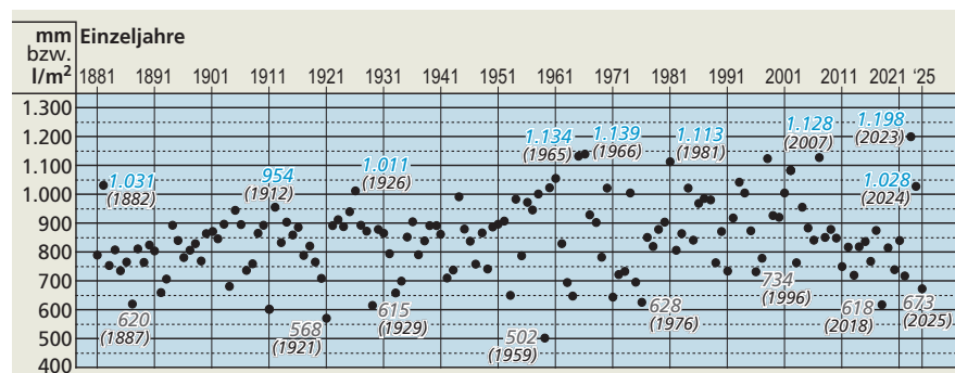
Abb. 2: Niederschläge in NRW in Einzeljahren
