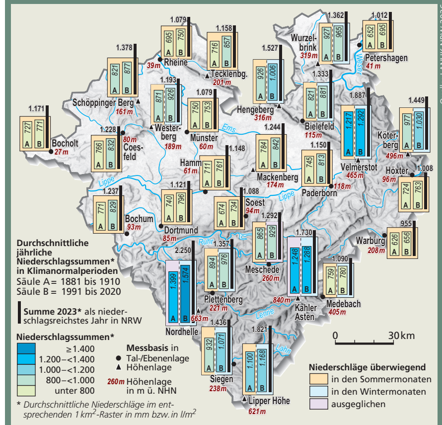
Abb. 3: Jährliche Niederschläge in Klimanormalperioden sowie Niederschläge 2023 in Westfalen
