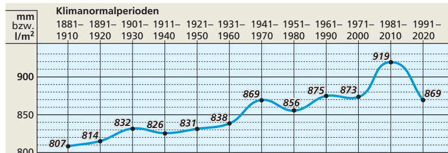
Abb. 1: Jährliche Niederschläge in NRW in Klimanormalperioden
