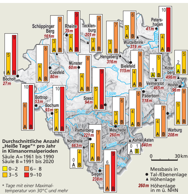
Abb. 4: Anzahl der heißen Tage in Klimanormalperioden in Westfalen
