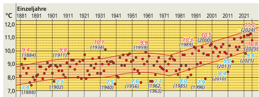
Abb. 2: Durchschnittstemperaturen in NRW in Einzeljahren
