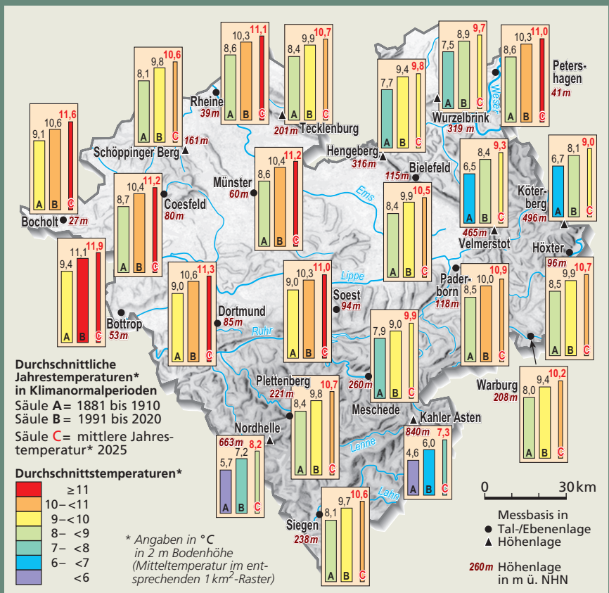
Abb. 3: Durchschnittstemperaturen in Klimanormalperioden sowie Jahrestemperaturen 2025 in Westfalen
