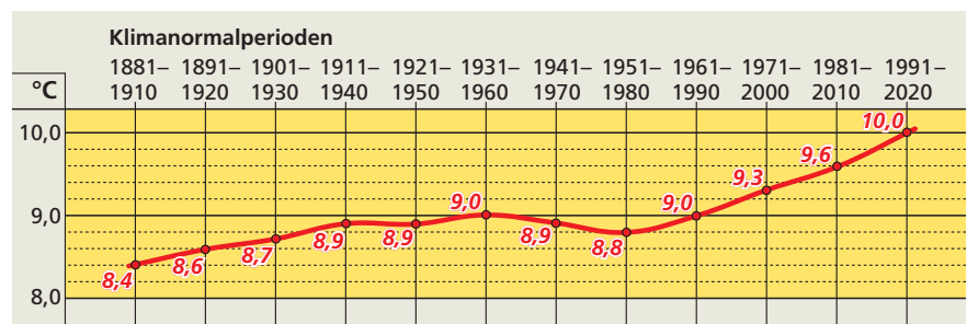
Abb. 1: Durchschnittstemperaturen in NRW in Klimanormalperioden
